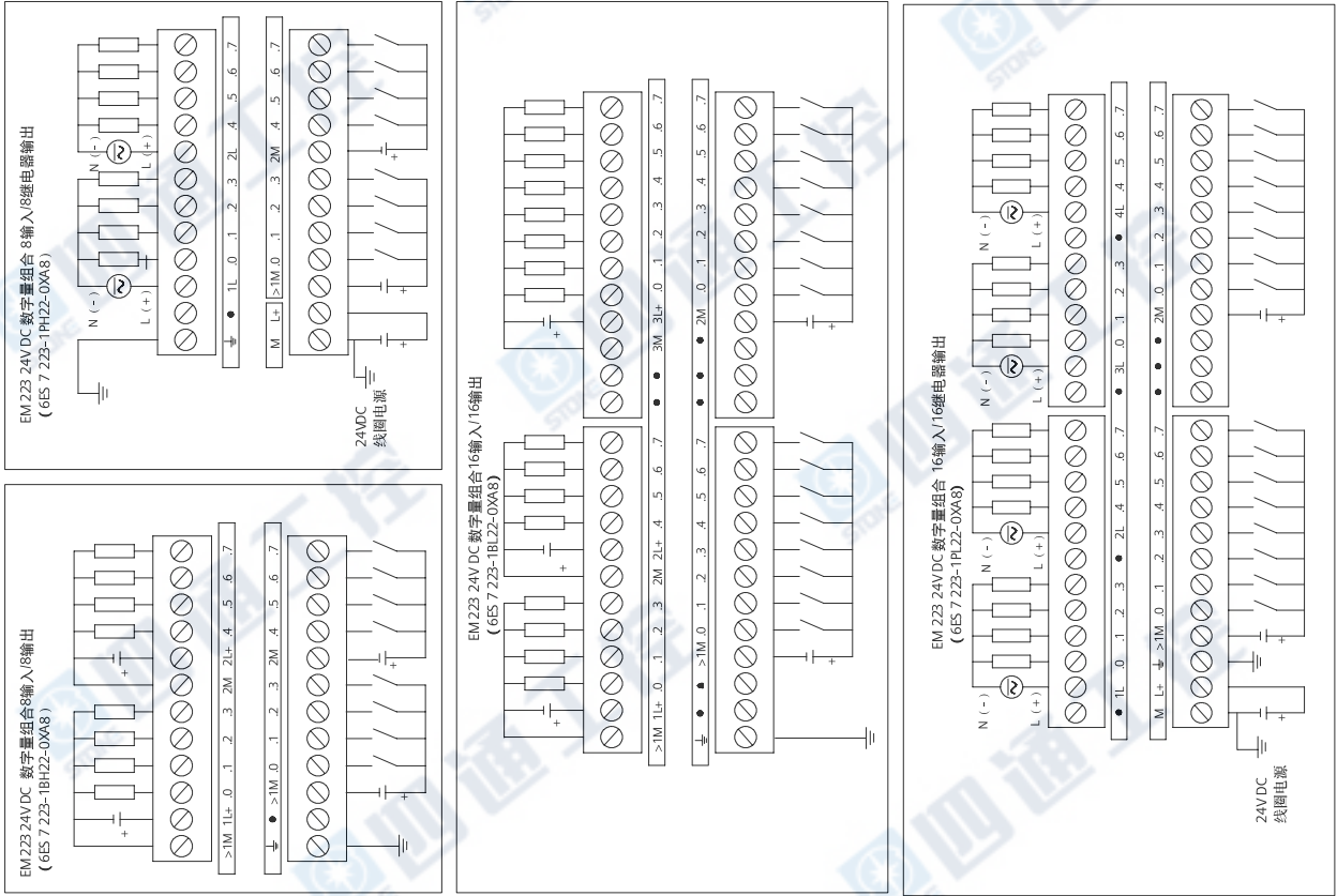
接线图
